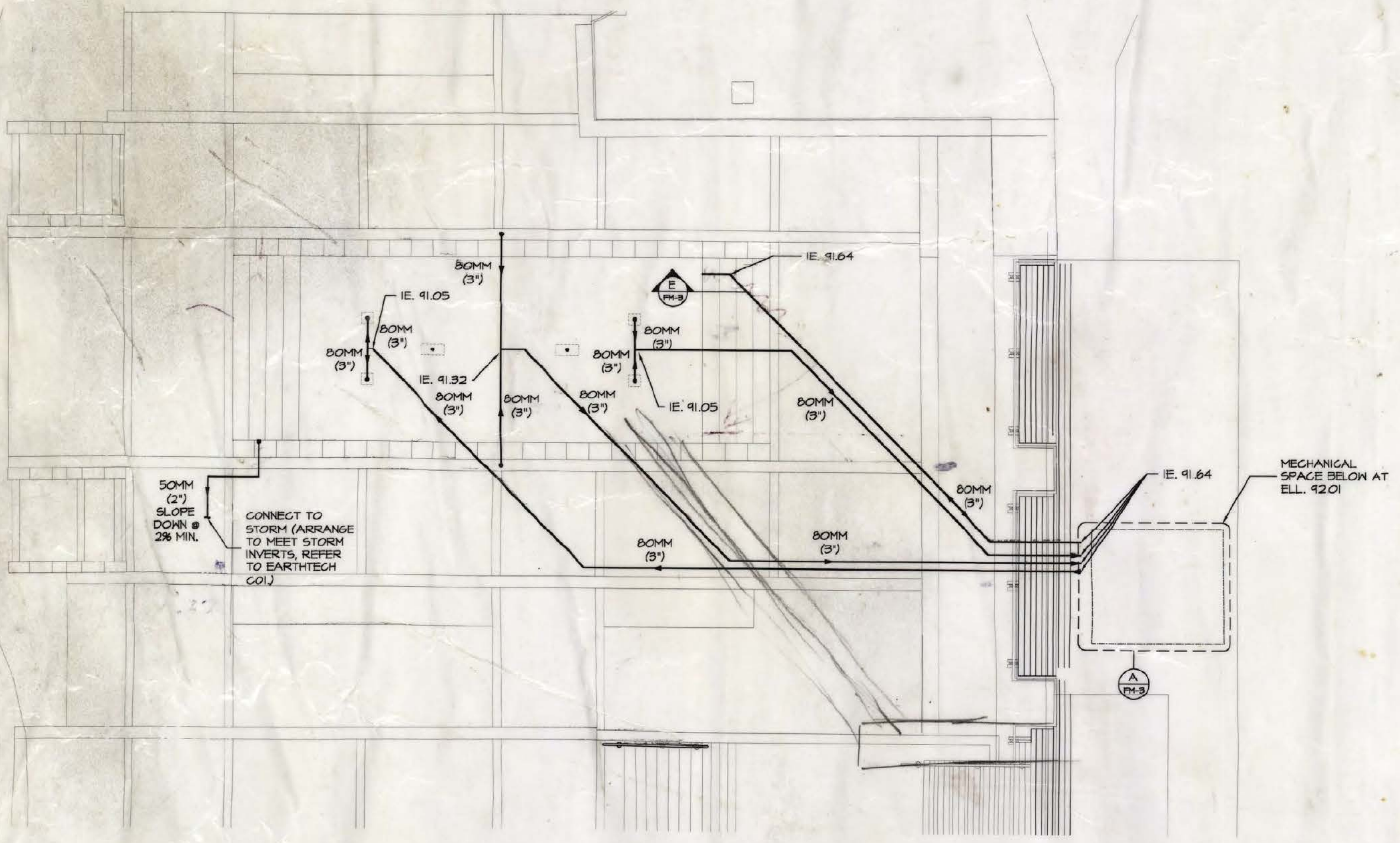
2 PIPING PLAN SCALE: 1:100
