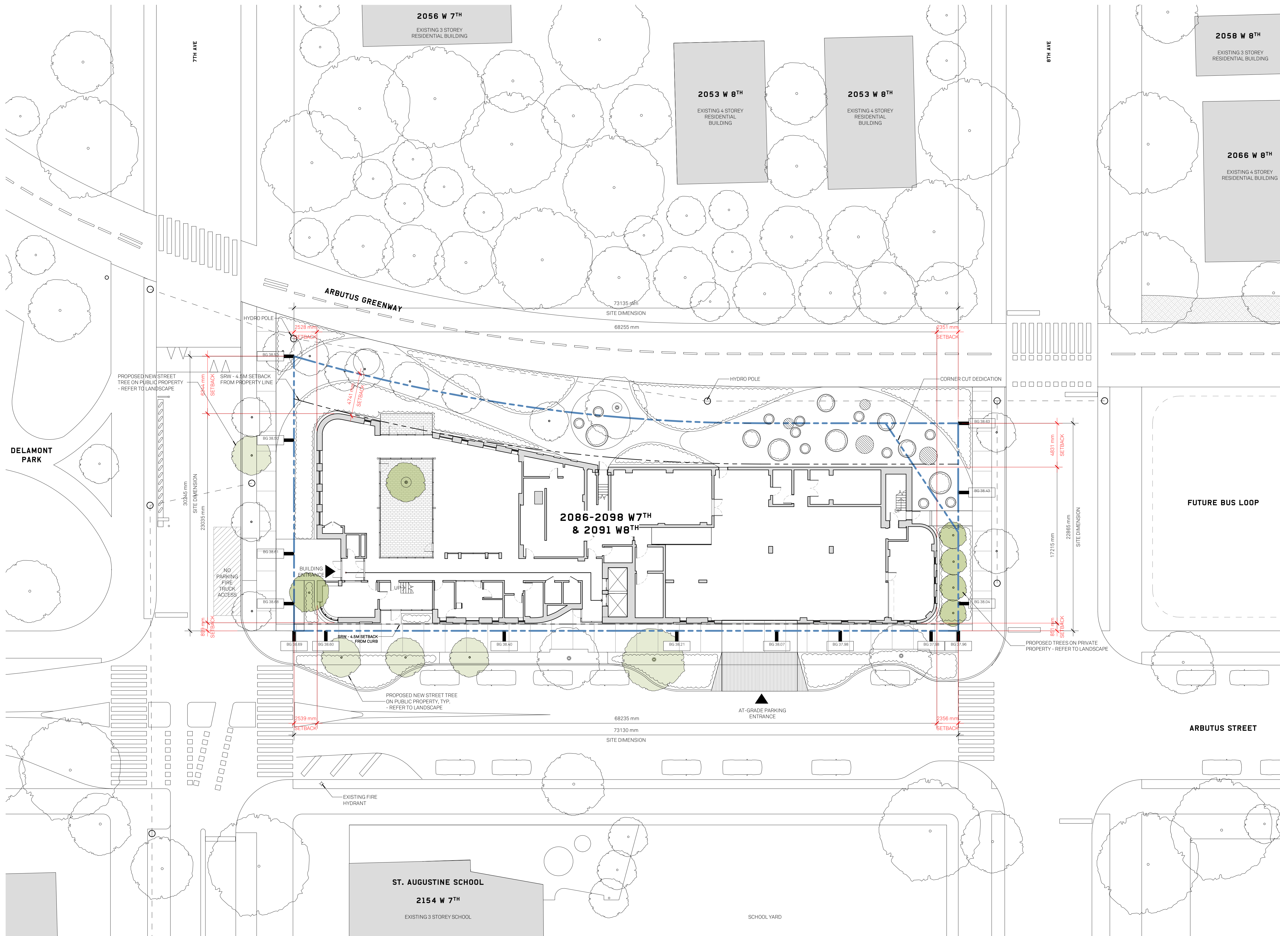
Site Plan 1:200
