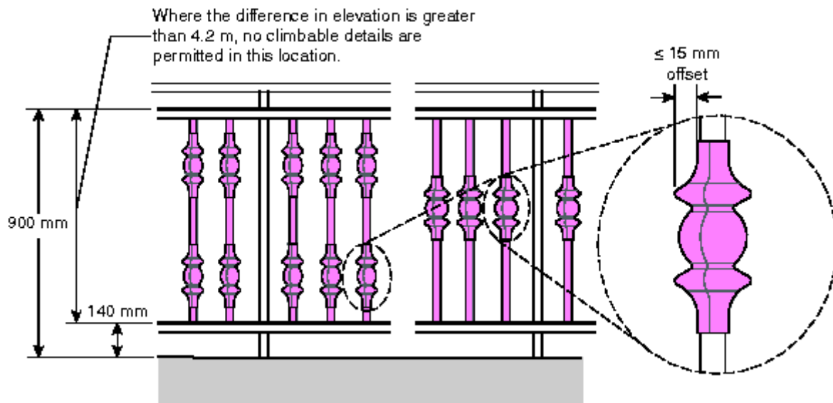
Figure A-9.8.8.6(1)-B
